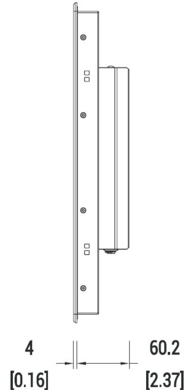
Seitenansicht
