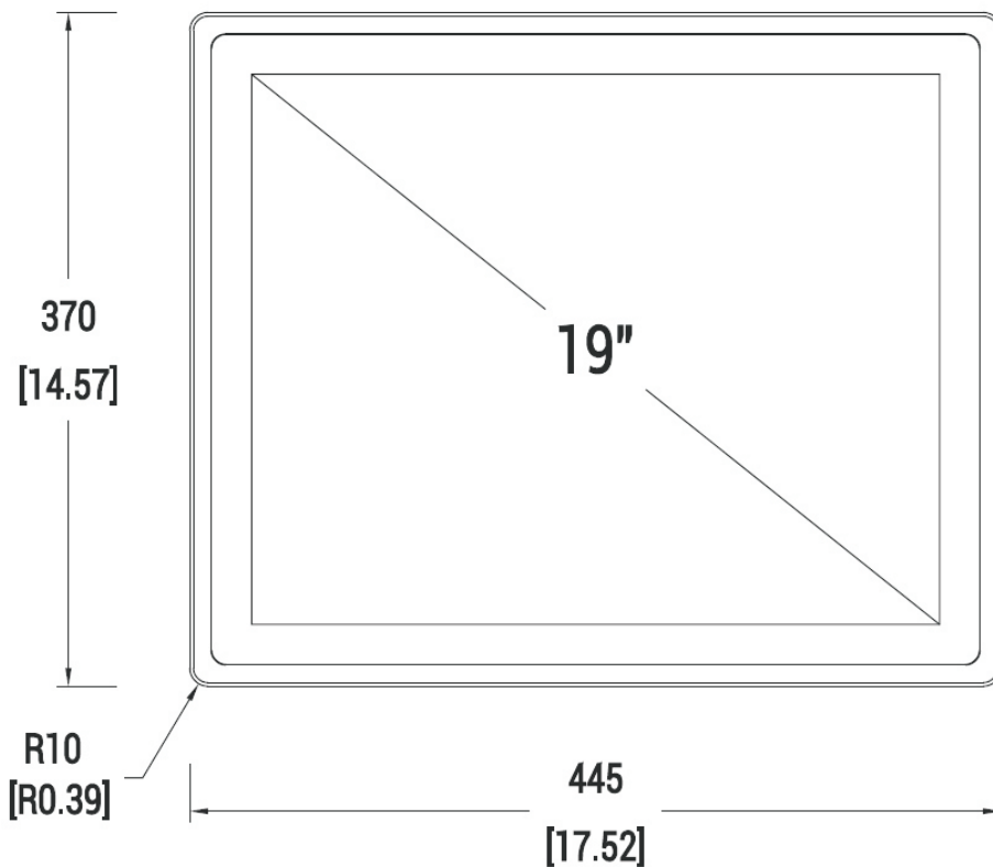
Frontansicht
