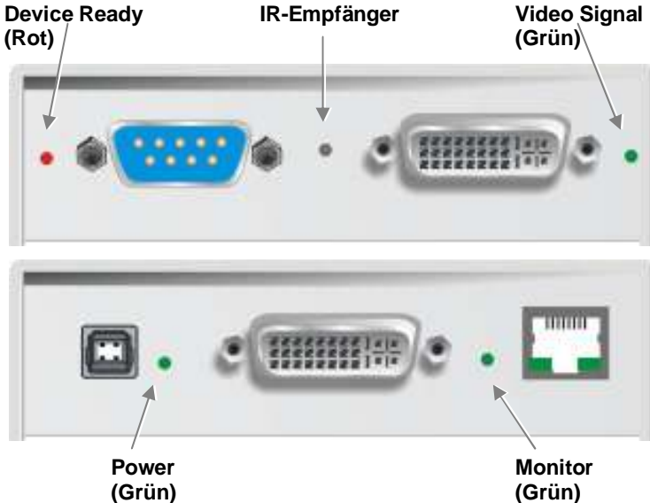
Bild 5 Diagnose- LEDs am RGB nach DVI(VGA) Konverter
