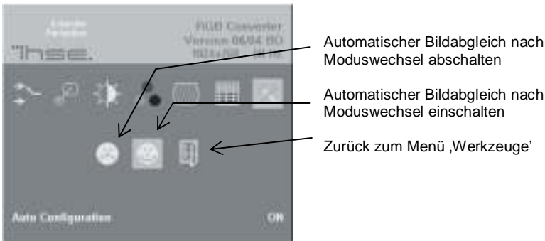
Bild 17 Untermenü 'Automatischer Bildabgleich'
