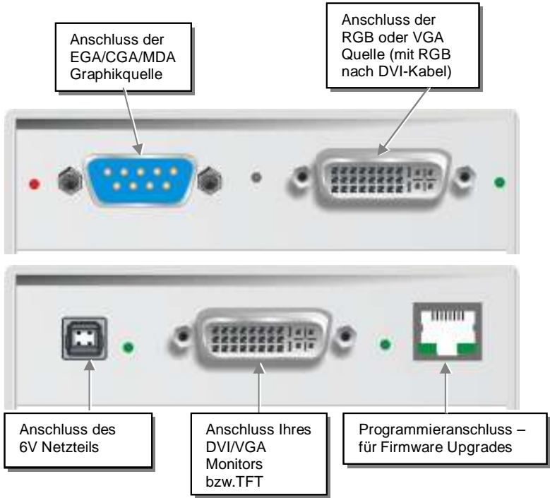
Bild 2 RGB nach DVI/(VGA) Konverter
